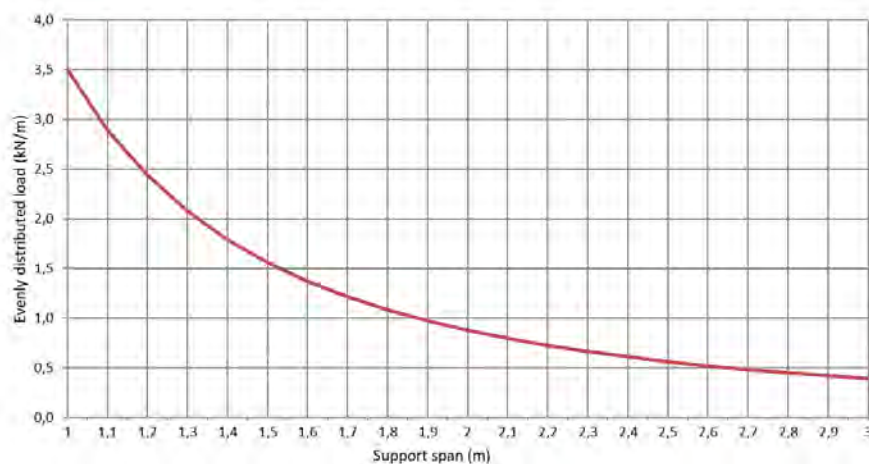
Permissible load KP 60/500 d=0,9mm (kN/m)
