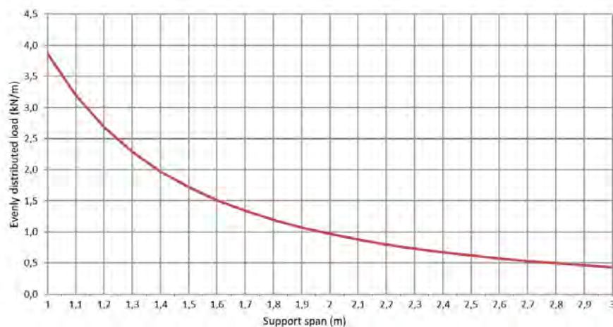
Permissible load KP 60/600 d=0,9mm (kN/m)
