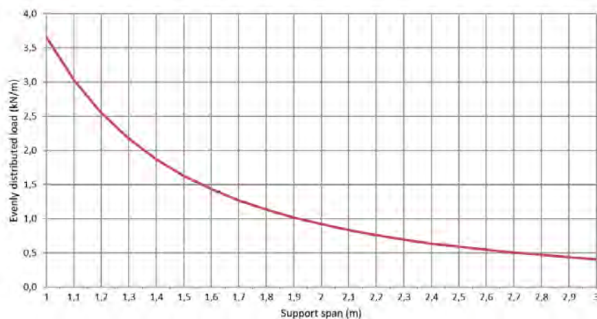
Permissible load KP 60/200 d=0,8mm (kN/m)
